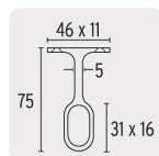
Medidas (mm)
