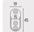
Medidas (mm)
